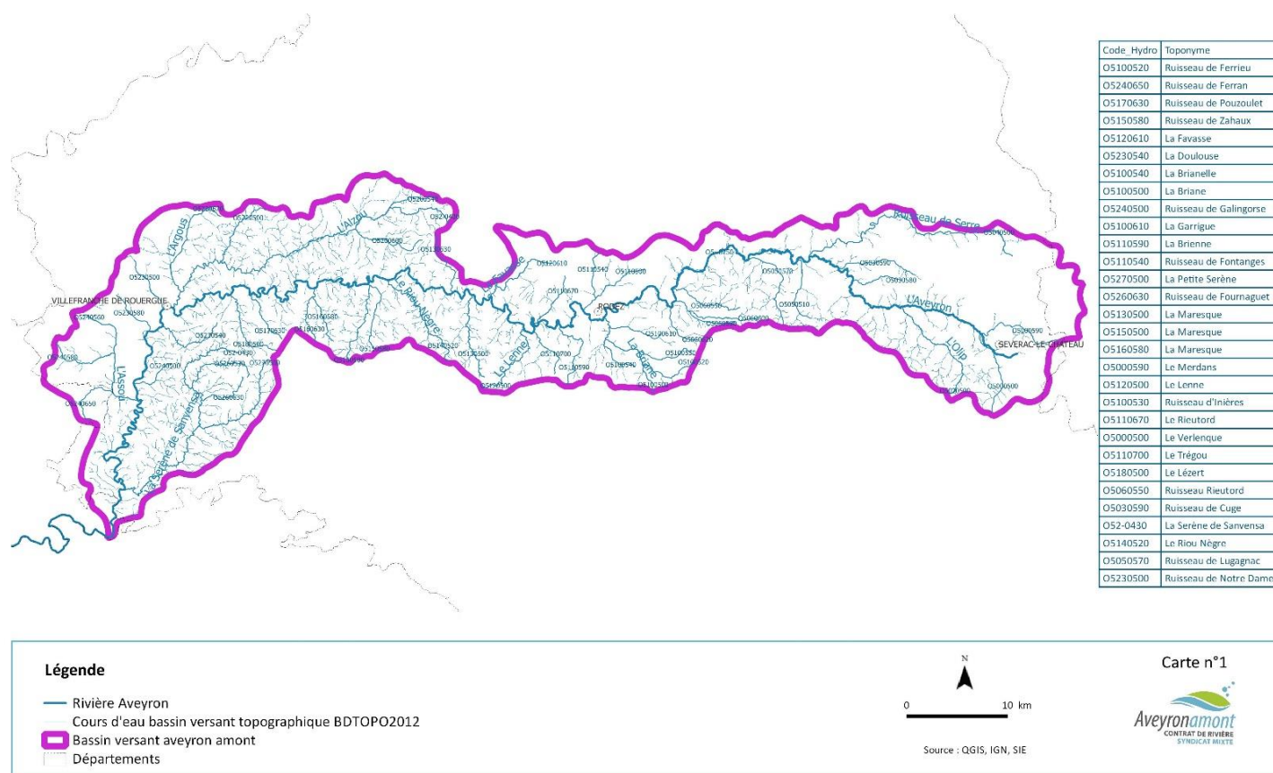
Atlas Cartographique Carte n° 1 : Les cours d'eau du bassin versant Aveyron Amont
